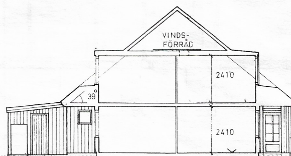
SEKTION
