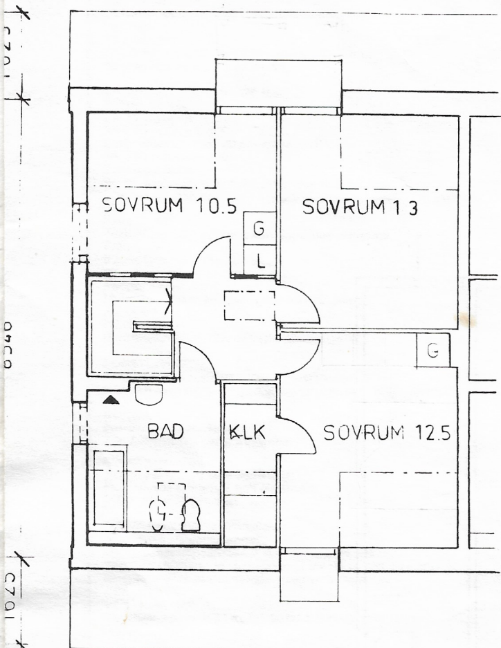
ÖVERPLAN
